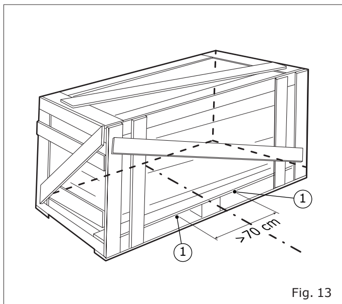
1. Punti di sollevamento
