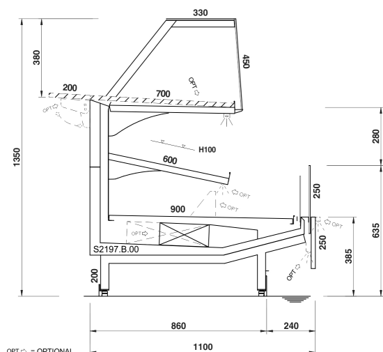
Sezione Cross Over Impact H1350_REF-NEUTRO
