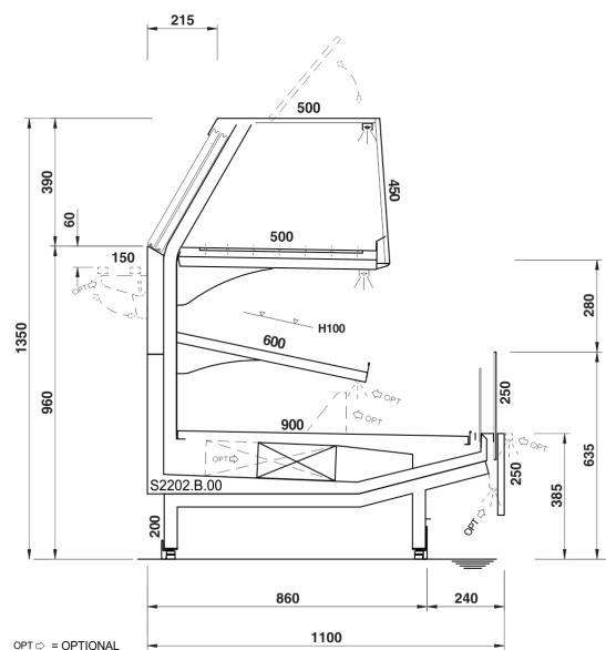
Sezione Cross Over Impact H1350_REF-HOT
